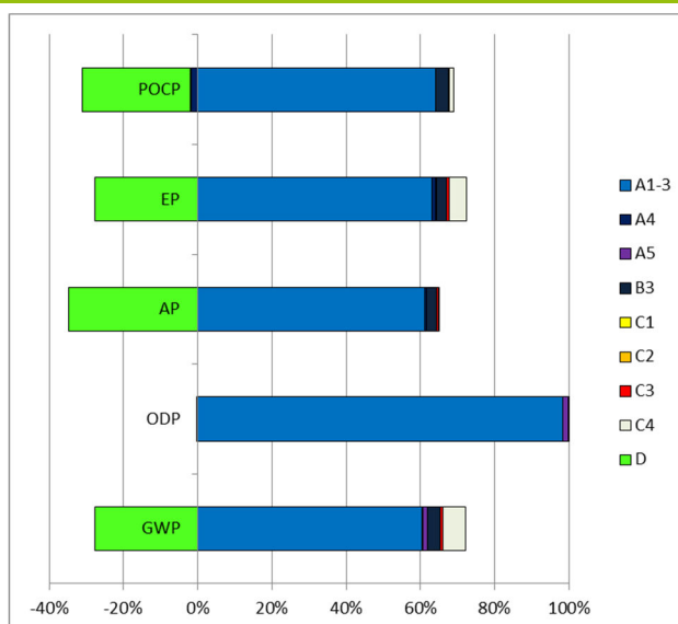
Abbildung 2: Sektionaltore
